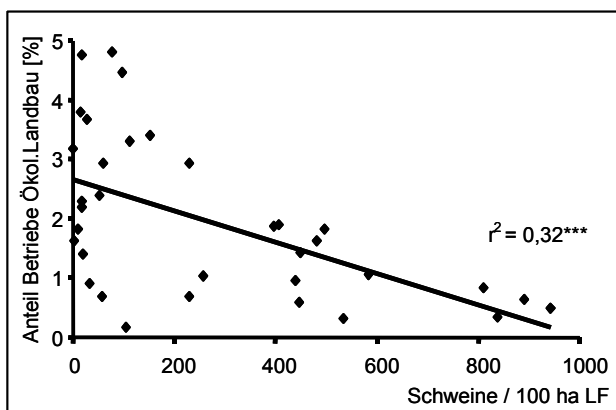
Abbildung 4. Beziehung zwischen Dichte an Schweinen und Anteil ökologisch wirtschaftender Betriebe in den Landkreisen NRW (n = 34)
