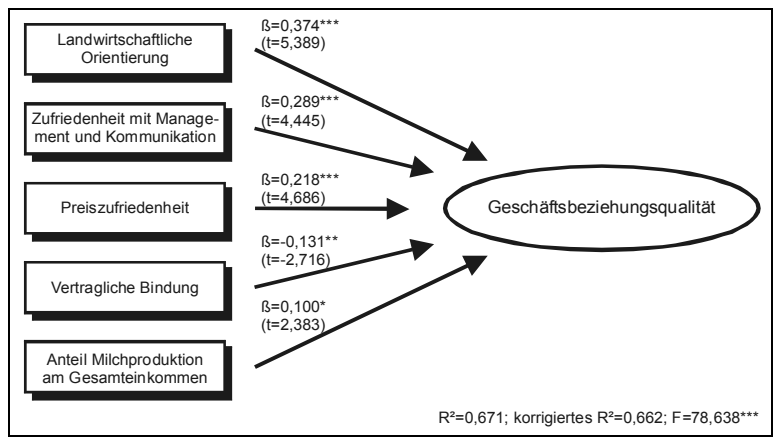
Abbildung 9. Regressionsmodell
